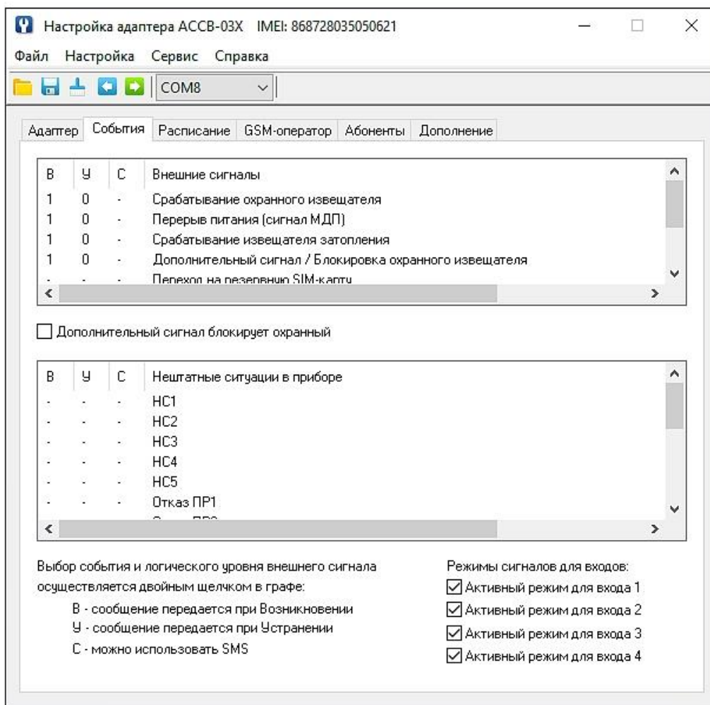
Рис.7. Вкладка «События» программы «Настройка адаптера АССВ-03Х».
