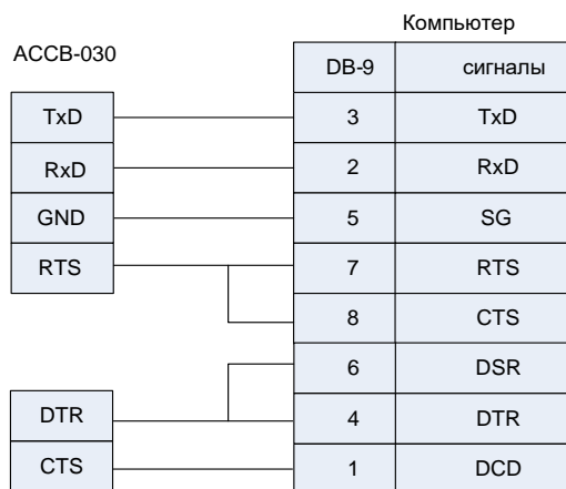
Рис.9. Схема подключения АССВ-030 к компьютеру в качестве универсального модема.
