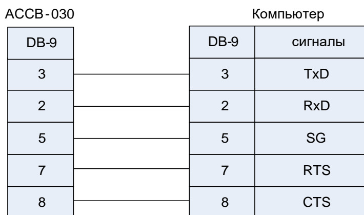
Рис.5. Подключение АССВ-030 к компьютеру при настройке.
